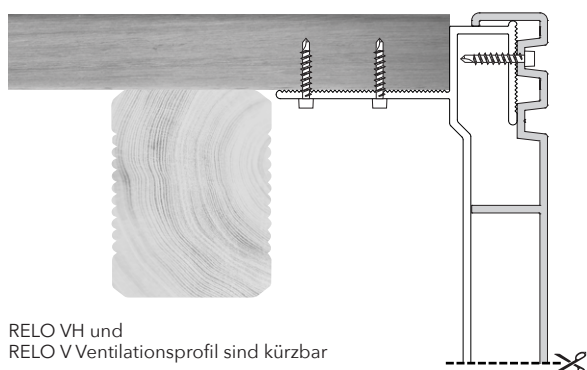
RELO VH ist variabel für Dielenstärken von 20 - 42 mm
